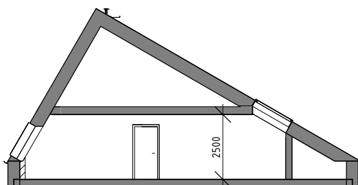
PRINCIPSEKTION 1:200
